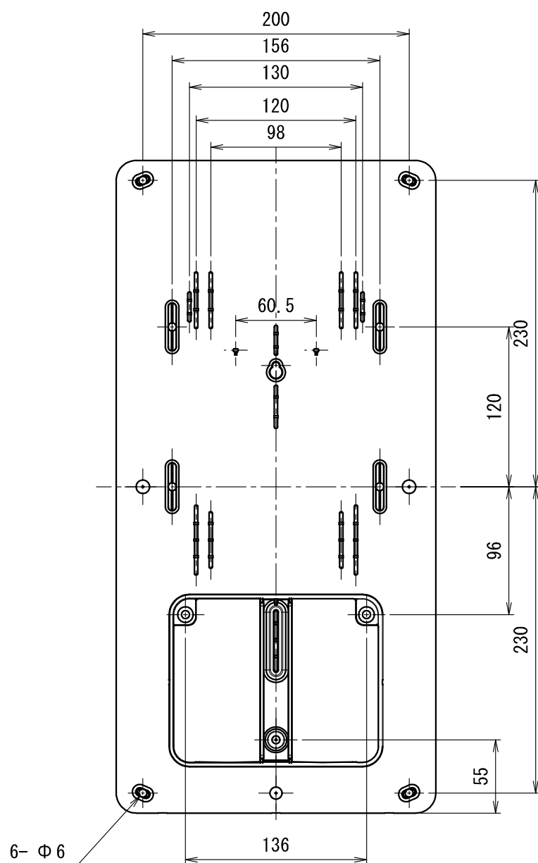
差込通線用フックアウト (MD40, 70兼用)
