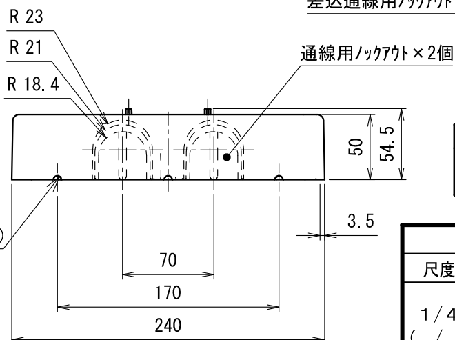
差込通線用フックアウト (MD40, 70兼用)
